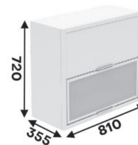
Aéreo 810MM com 2 Portas Cinamomo / Connect - 8198085 Cinamomo / Grafite - 8198084 Cinamomo / Off White - 8198087 M²: 0,0435 Volume: 01
